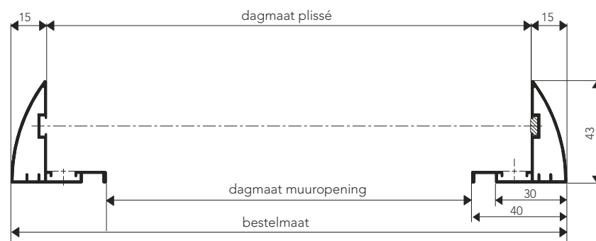
Bovenaanzicht (doorsnede)
