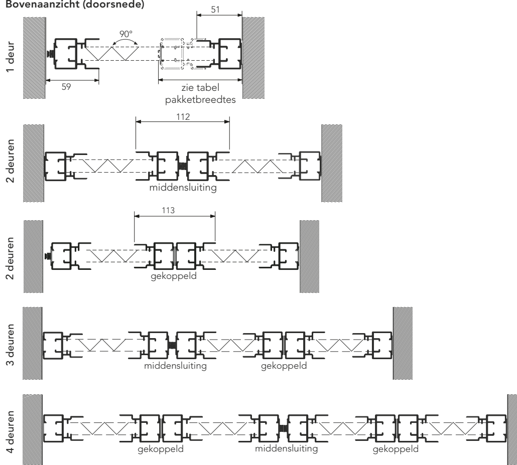
Bovenaanzicht (doorsnede)
