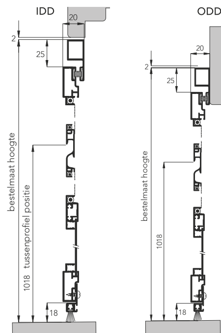
Zijaanzicht IDD en ODD (doorsnede)
