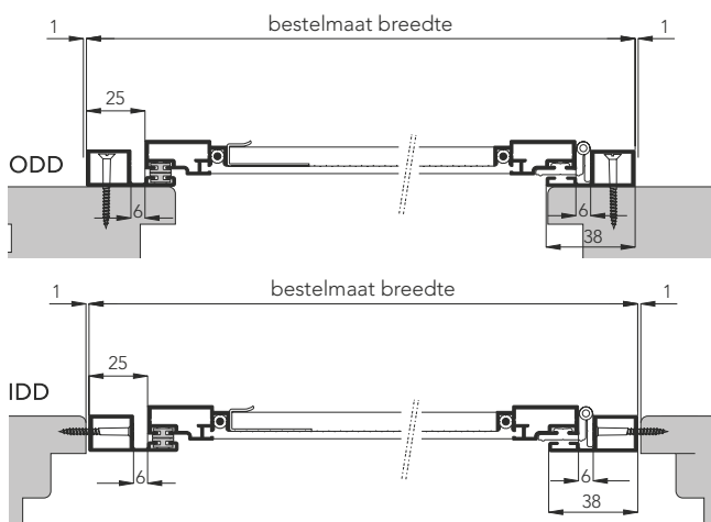
Bovenaanzicht ODD en IDD (doorsnede)
