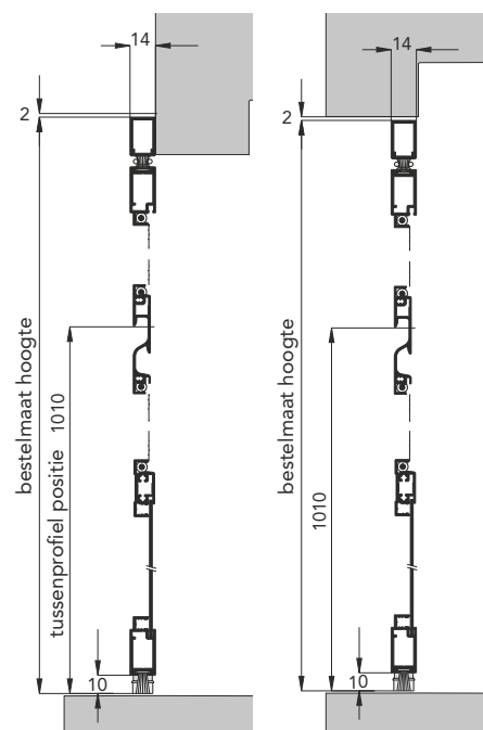
Zij aanzicht (doorsnede)
