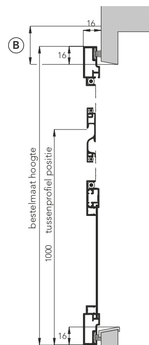
Zij aanzicht (doorsnede)
