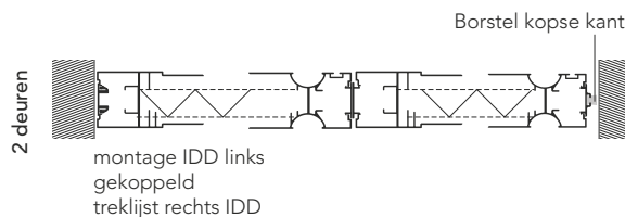
montage IDD links + rechts middensluiting treklijst IDD
