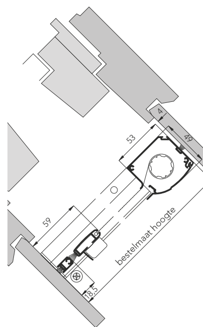
Zijaanzicht (doorsnede)
