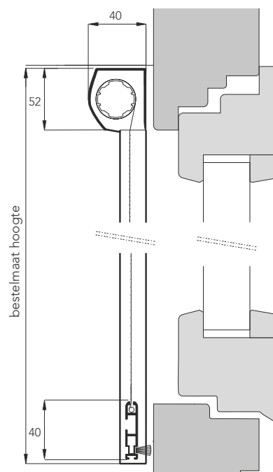
Zijaanzicht (doorsnede)
