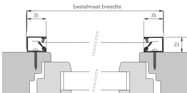
Bovenaanzicht (doorsnede)
