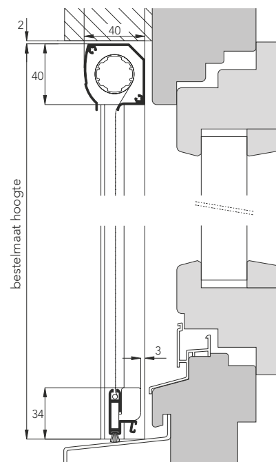
Zijaanzicht (doorsnede)
