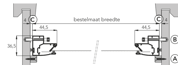
Bovenaanzicht (doorsnede)
