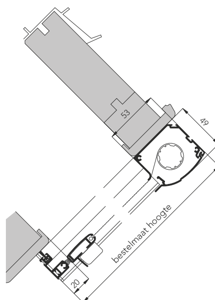
Zijaanzicht (doorsnede)
