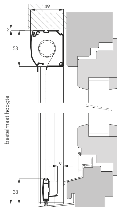
Zijaanzicht (doorsnede)
