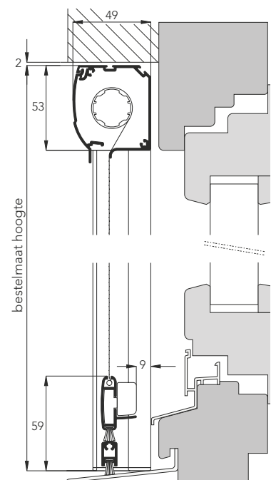
Zijaanzicht (doorsnede)
