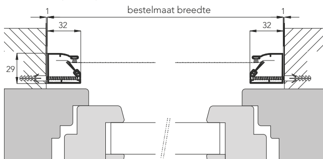
Bovenaanzicht (doorsnede)
