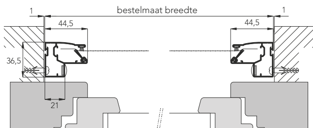
Bovenaanzicht (doorsnede)
