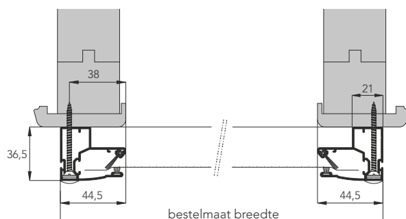
Bovenaanzicht (doorsnede)
