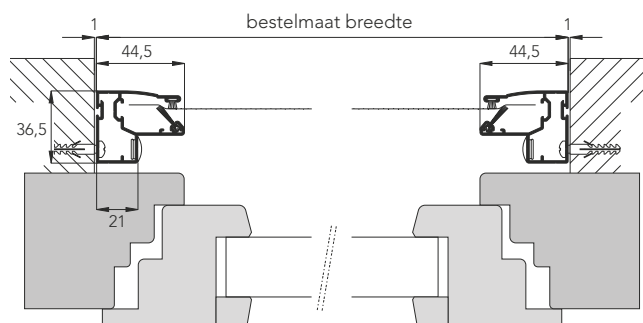
Bovenaanzicht (doorsnede)
