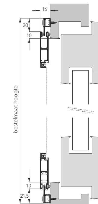
Zijaanzicht (doorsnede)
