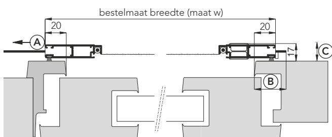
Bovenaanzicht (doorsnede)
