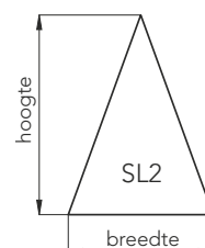
Gelijkbenige driehoek
