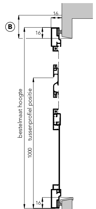
Zij aanzicht (doorsnede)
