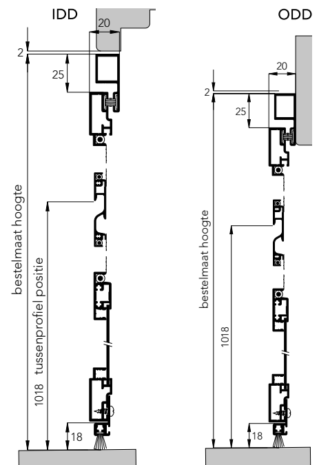
Zijaanzicht IDD en ODD (doorsnede)
