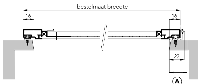
Bovenaanzicht (doorsnede)
