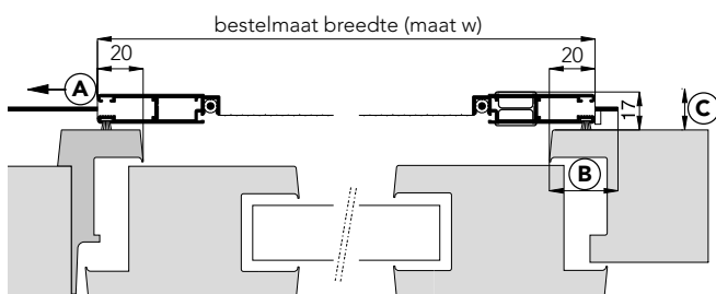
Bovenaanzicht (doorsnede)
