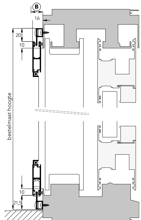
Zijaanzicht (doorsnede)
