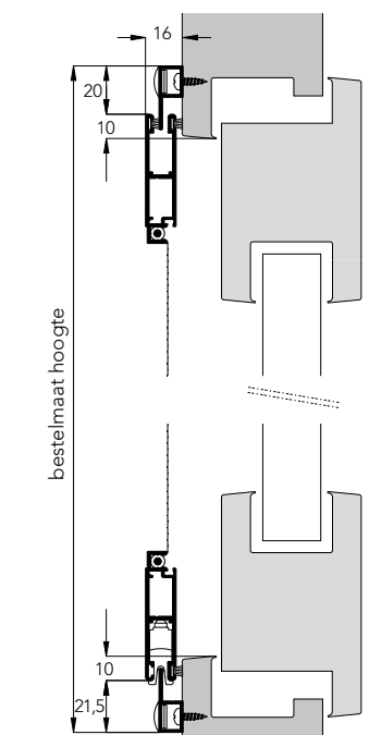
Zijaanzicht (doorsnede)
