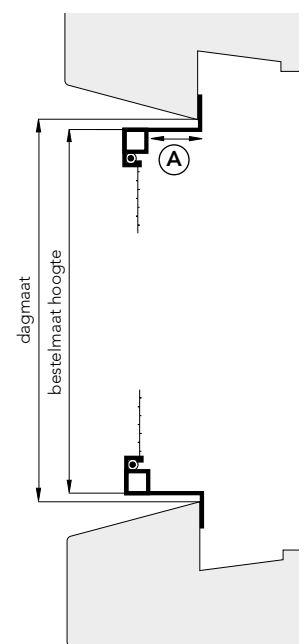
Zijaanzicht (doorsnede)
