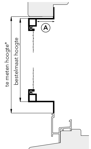
Zijaanzicht (doorsnede)
