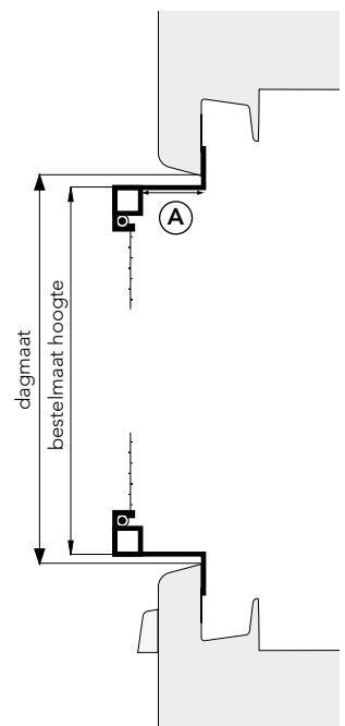
Zijaanzicht (doorsnede)
