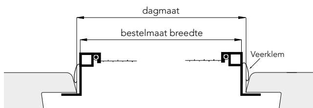
Bovenaanzicht (doorsnede)
